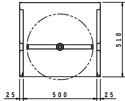
防火衣収納庫本体横断面
