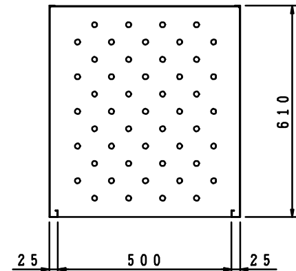
下段収納庫本体横断面
