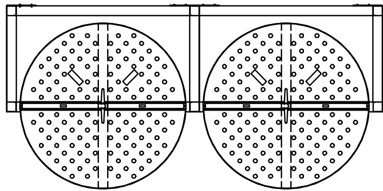
B-B断面図
