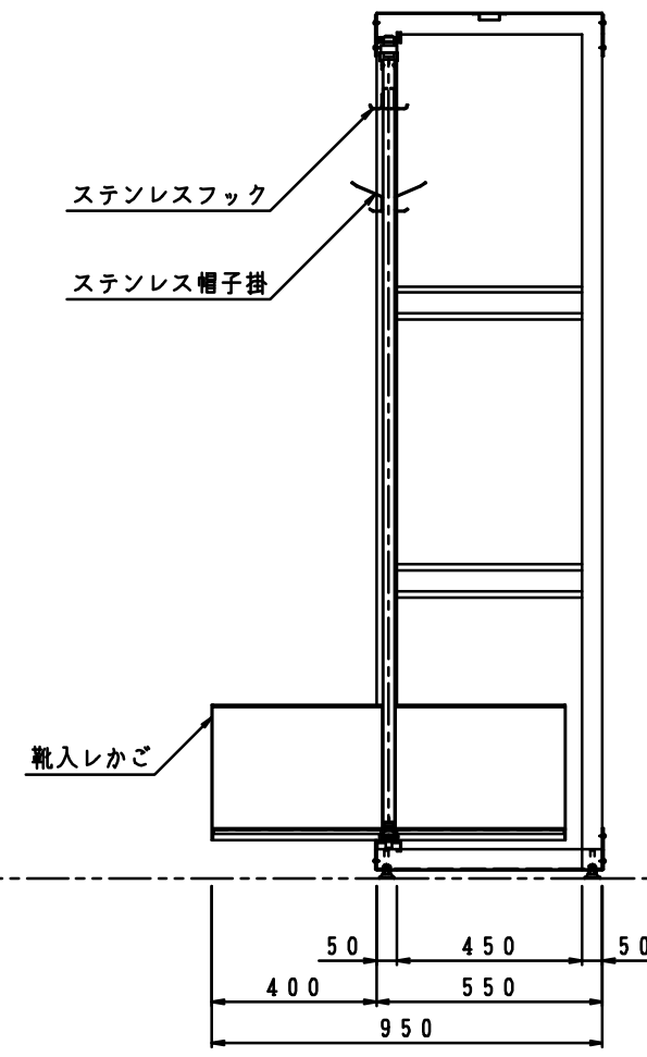
A-A断面図
