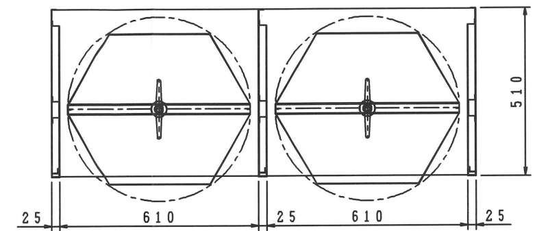
防火衣収納庫本体横断面
